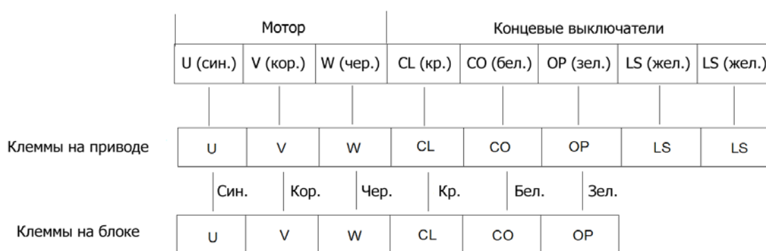
Рис. 5. Схема подключения привода
